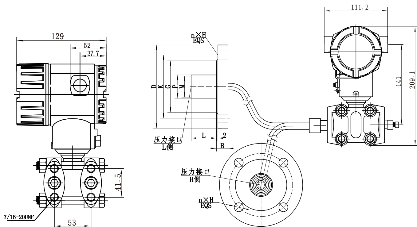
远传固定法兰插入筒 + 远传固定法兰插入筒带显示整机尺寸图 (不带显示尺寸与带显示一致)
